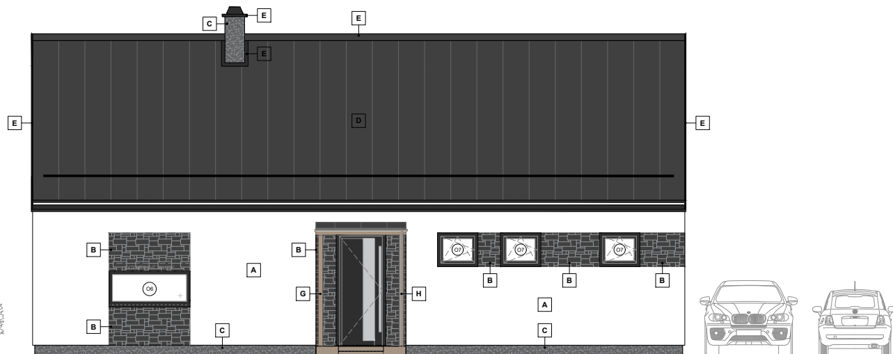
POHĽAD VÝCHODNÝ
