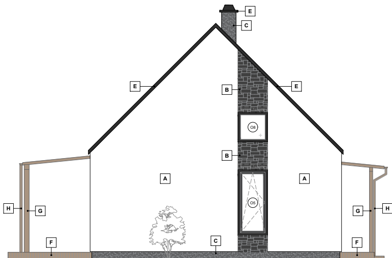
POHĽAD JUŽNÝ
