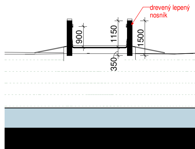
REZ A-A'
