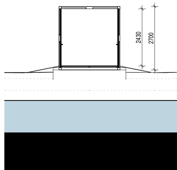
REZ A-A'
